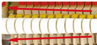
그랜드 피아노의 고음부터 저음에 걸친 해머의 크기 차이
