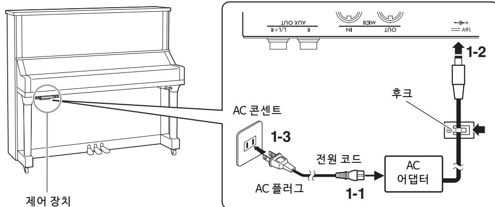
DC IN 잭이 후면에 없는 피아노:
