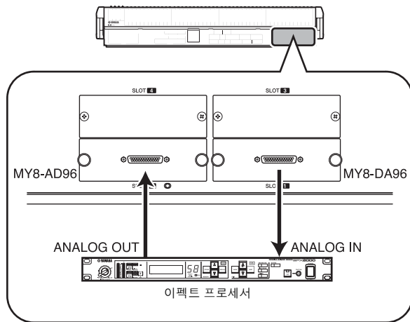
인서트 연결 예 ②
