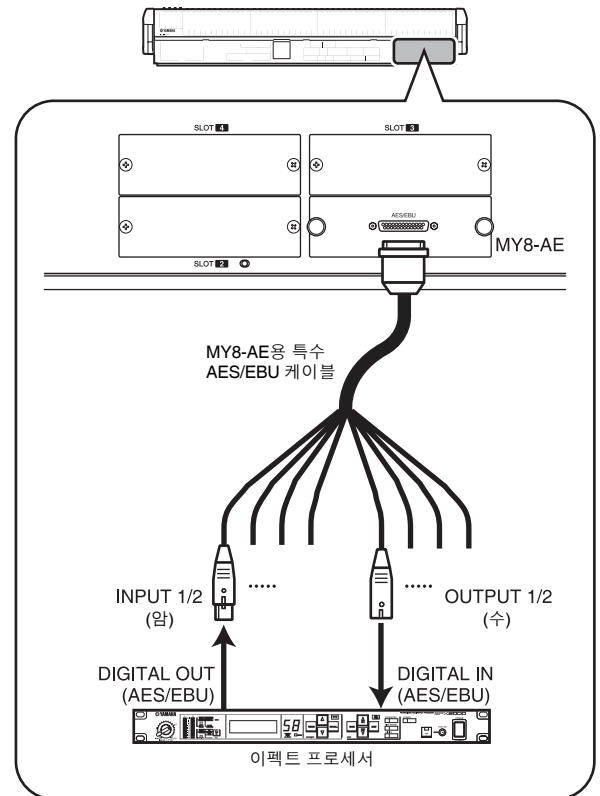
인서트 연결 예 ③
