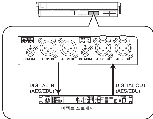
인서트 연결 예 ①
